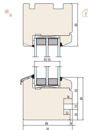
SYSTEM NATURO 92-Fix Innere Fensterbankkräsung
