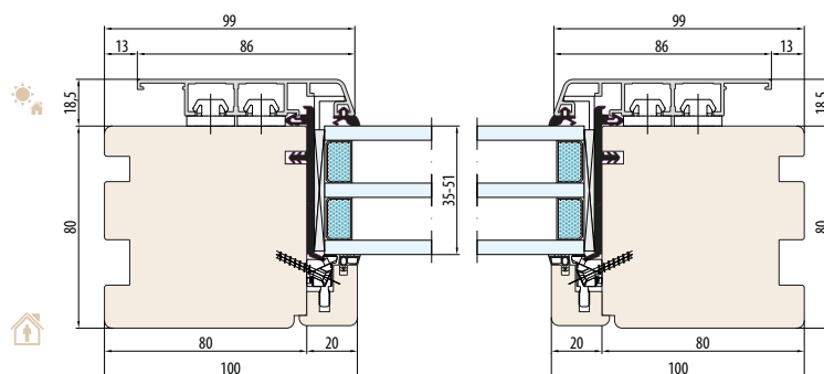
HORIZONTALSCHNITT B-B
