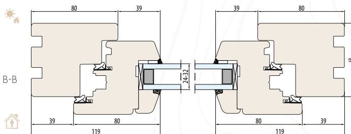
SYSTEM NATURO 68 Äußere Fensterbankfräsung
