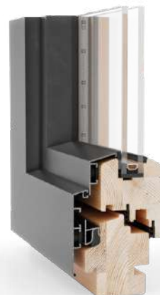
Profil Reno Line (mit Fensterbankfräsung)
