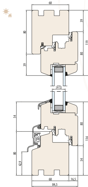
SYSTEM NATURO 68 Ohne Fensterbankfräsung
