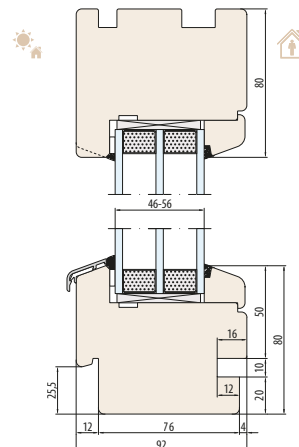
SYSTEM NATURO 92-Fix Innen- und Außenfensterbankkräsung
