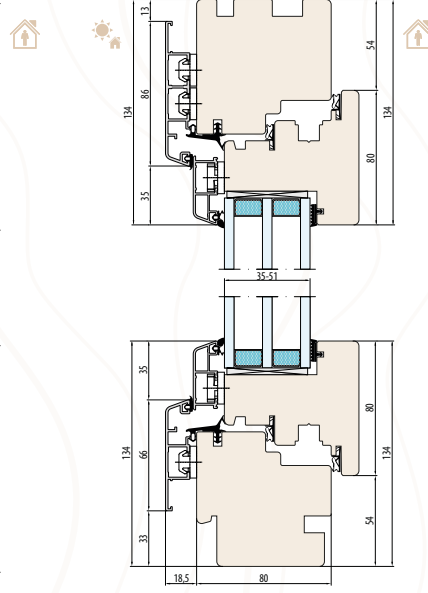
SYSTEM NATURO 80 ALU GEMINI CLASSIC Innen- und Außenfensterbankfräsung
