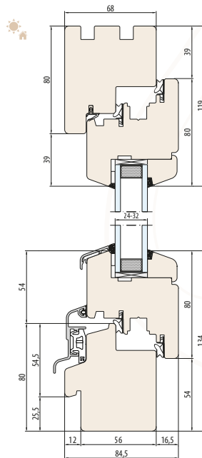
SYSTEM NATURO 68 Äußere Fensterbankfräsung
