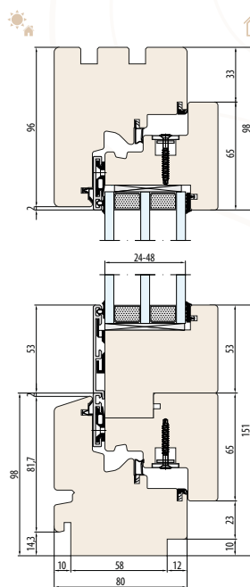
SYSTEM ESPERIA LIFE 80 Einfügelige Balkontüren mit hoher Schwelle
