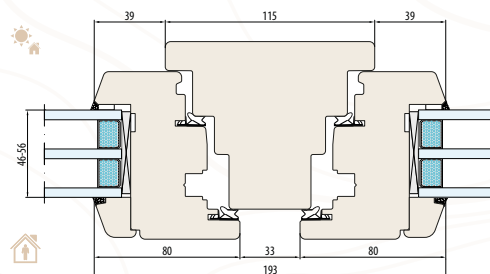
SYSTEM NATURO 92 Fester Pfosten 115 mm (Horizontalschnitt)
