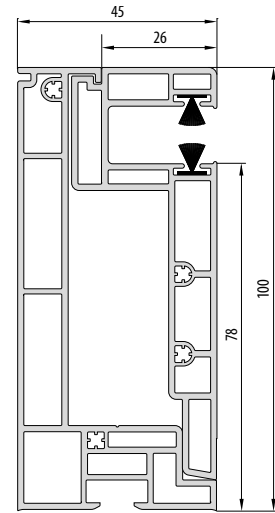
• PPRA12** • Styroterm Revision von außen
